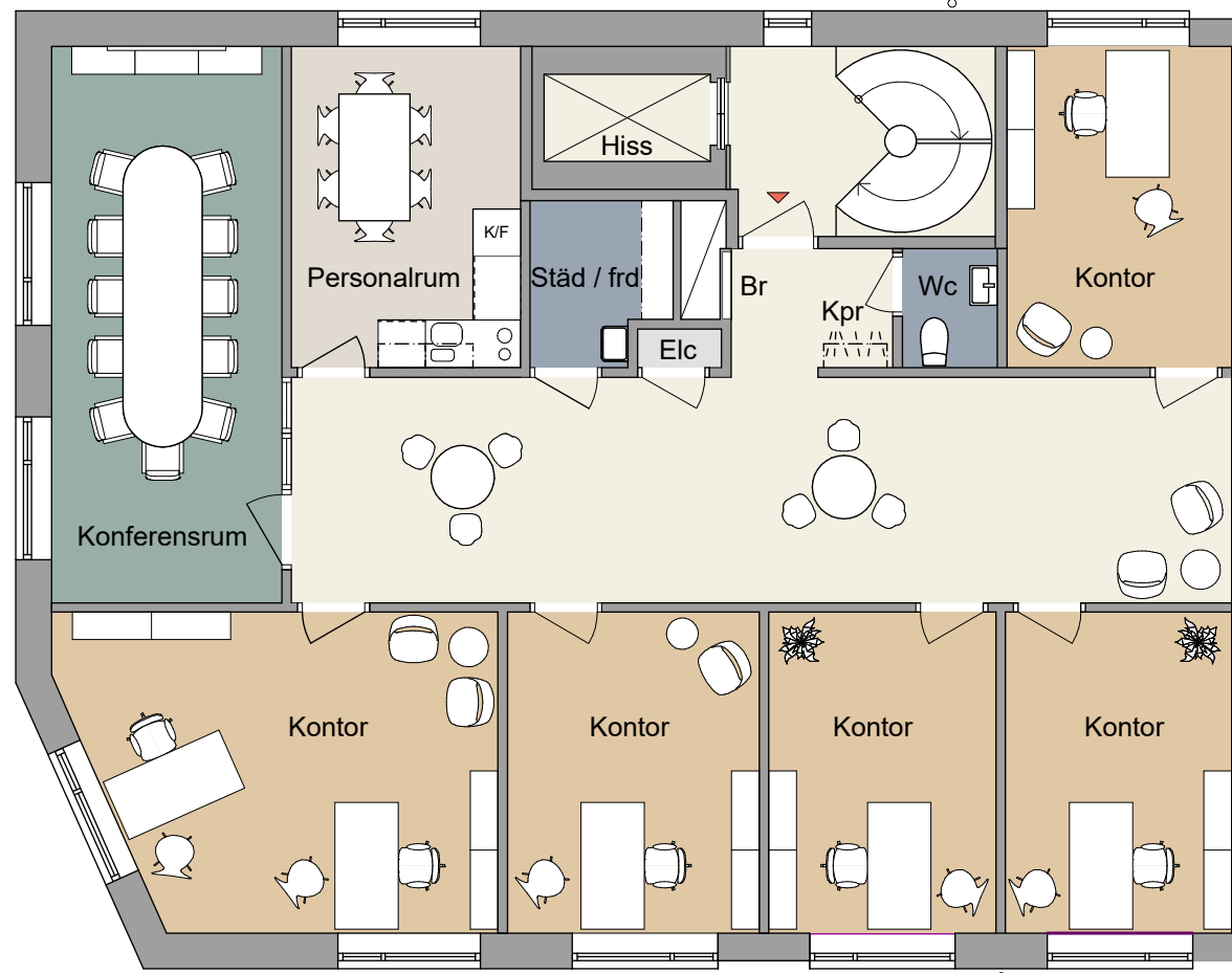
PLAN 4, VÅNING 2 TRAPPOR
